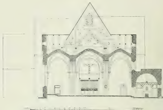
Fig. 23. Tvärsnitt av kyrkan, lagd genom tvärskeppet och Ragvald Knap-hövdes gravkor. Efter uppmätning av S. Curman o. A. Roland 1907, kompletterad av H. Sundberg 1927.
